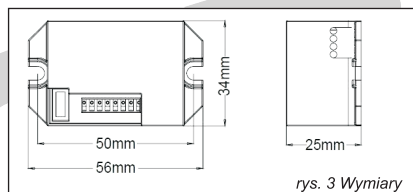
rys. 3 Wymiary
